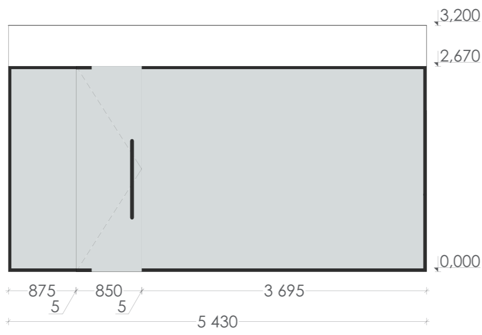
В-2 Скляна перегородка 1:50
