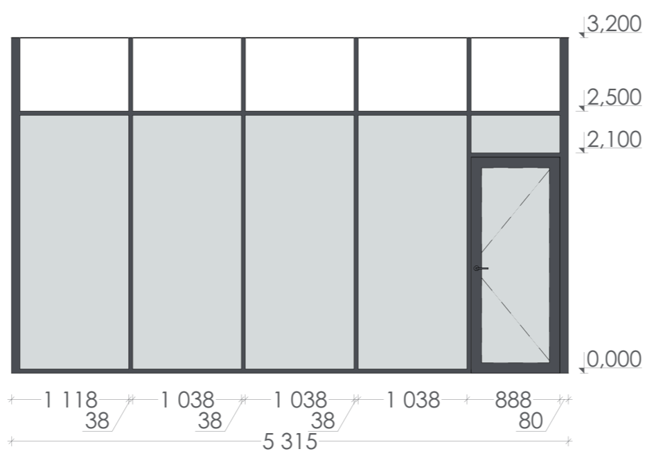
В-3 СП конструкція 1:50
